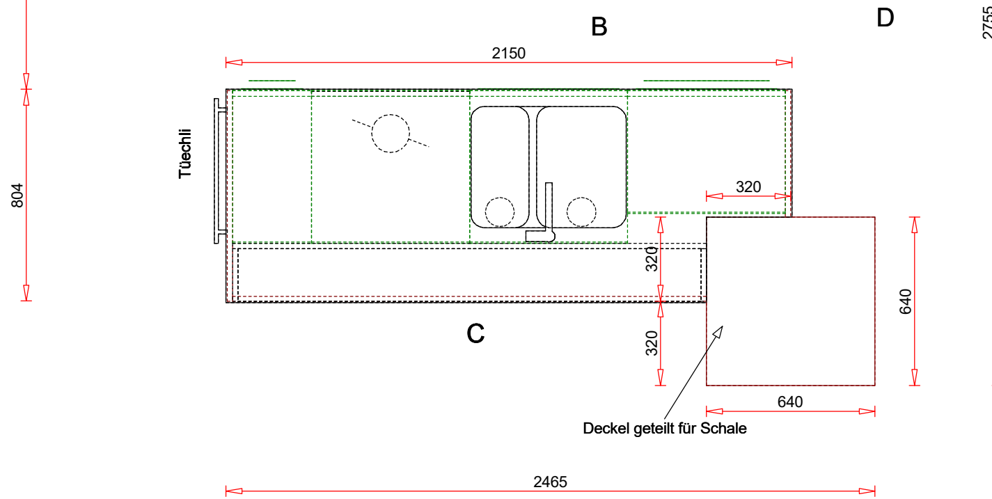
Grundriss
